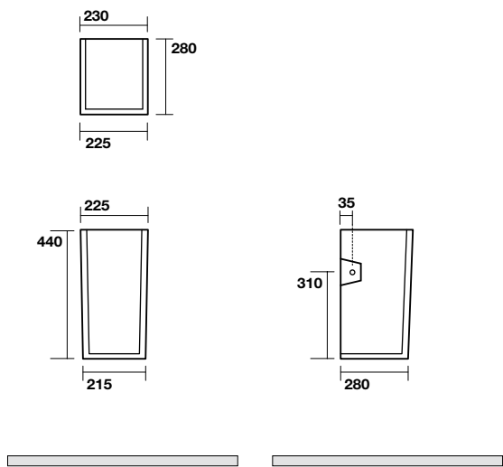
353701C Lavabo 45x25 sospeso o appoggio monoforo (centrale) One hole wall hung or free standing washbasin 45x25 (central)
