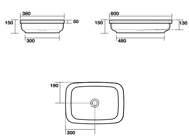
5143 Lavabo appoggio/incasso 60x38 Freestanding/inset washbasin 60x38
