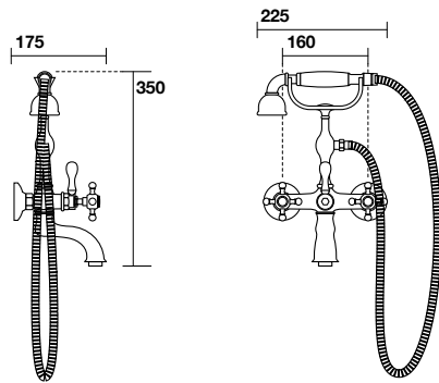
7394 Gruppo vasca esterno con doccia duplex Visible bath group with shower duplex
