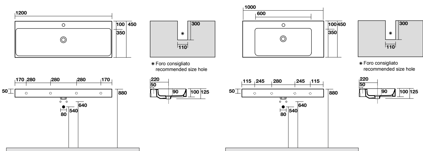
3534 Lavabo 120x45 sospeso, appoggio o su colonna monoforo One hole wall hung, counter top or on pedestal washbasin 120x45
