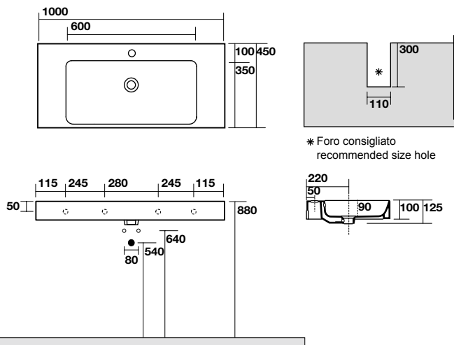
3550 Lavabo 100x45 sospeso, appoggio o su colonna monoforo One hole wall hung, counter top or on pedestal washbasin 100x45
