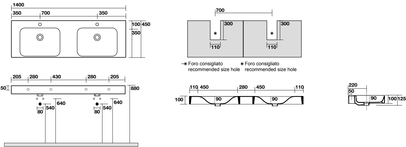
3536 Lavabo 140x45 doppia vasca sospeso, appoggio monoforo One hole wall hung or counter top double basin 140x45
