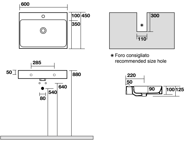
3531 Lavabo 60x45 sospeso, appoggio o su colonna monoforo One hole wall hung, counter top or on pedestal washbasin 60x45
