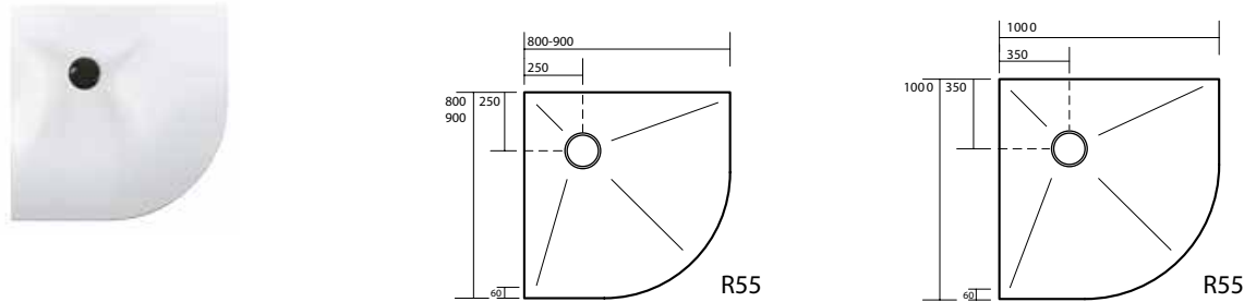
Piletta sifonata Ø 90 mm per piatti doccia Drain plug Ø 90 mm for shower trays
