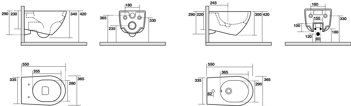
3714 Vaso sospeso NORIM completo di protezione acustica e antiurto Wall hung wc NORIM, sound and shock proof plate included 3724 Bidet sospeso monoforo completo di protezione acustica e antiurto One hole wall hung bidet, sound and shock proof plate included
