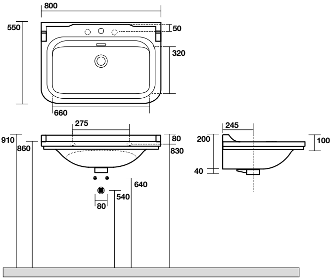
4141 Lavabo 80x55 sospeso o su colonna monoforo (tre fori a richiesta) One hole wall hung or on pedestal washbasin 80x55 (three holes on demand)
