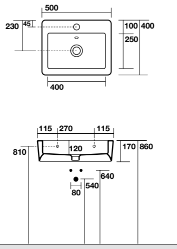
3250 Lavabo 70x43 sospeso o appoggio monoforo One hole wall hung, or free standing washbasin 70x43
