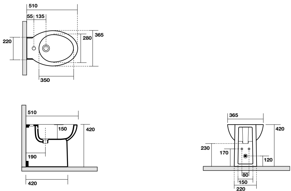
4440 Lavabo 62 appoggio o su colonna monoforo One hole counter top or on pedestal washbasin 62
