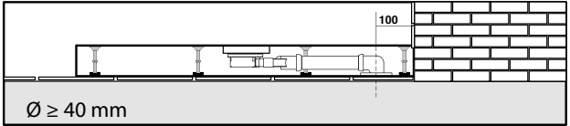
istallazione in appoggio free standing shower tray
