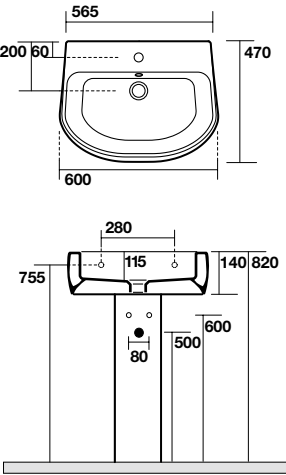
4546 Lavabo 60x47 sospeso, appoggio o su colonna monoforo One hole wall hung, counter top or on pedestal washbasin 60x47 4570 colonna pedestal
