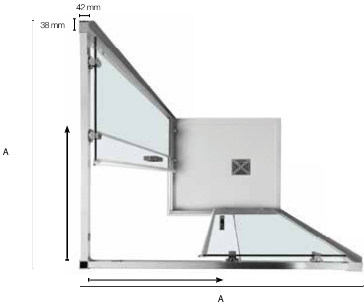
Versione angolare DX Right corner version
