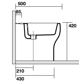
4520 Bidet monoforo 50 cm Btw one hole bidet 50 cm
