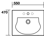
3942 Lavabo incasso monoforo 55x47xH.2 (3 fori a richiesta) (4 lati smaltati) One hole inset basin 55x47xH.2 (3 holes on demand) (4 glazed sides)
