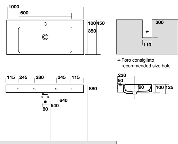
3550 Lavabo 100x45 sospeso, appoggio o su colonna monoforo One hole wall hung, counter top or on pedestal washbasin 100x45
